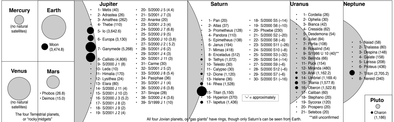
Mercury Venus Earth Moon Mars Jupiter Saturn Uranus Neptune Pluto Sun
